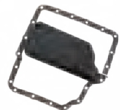
Filtro Transmisión Auto. JF506E/VW09A 5 Velocidades Golf 1.8 4cil. Jetta 2.0L 4cil. 00-05 Bora 1.8-1.9L 4cil. 02-07 OEM #09A-325-429 con Cuello 16mm Alto
